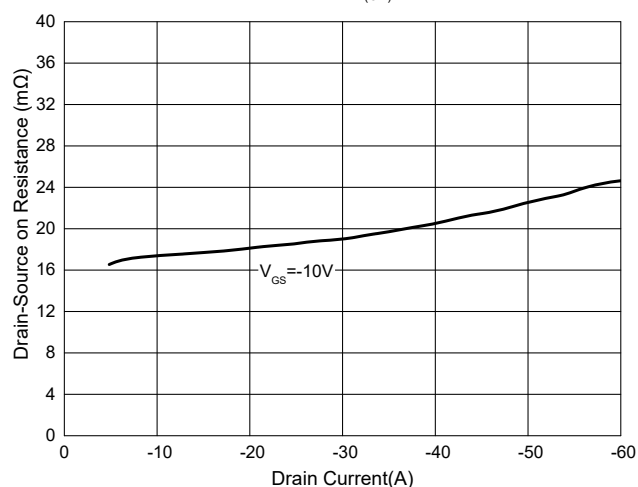
Fig. 7 - R_{DS(ON)} - I_D
