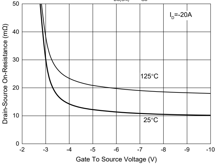
Fig. 3 - R_{DS(ON)} - V_{GS}
