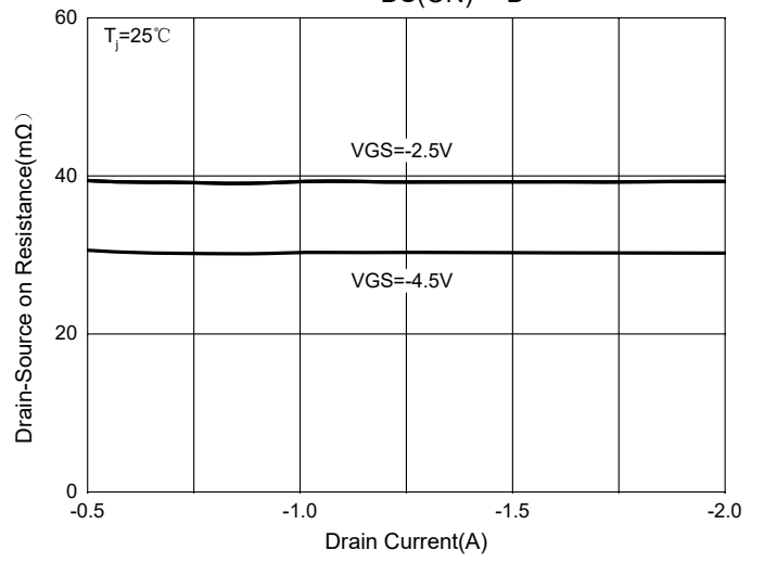
Fig. 4 - R_{DS(ON)} - I_D
