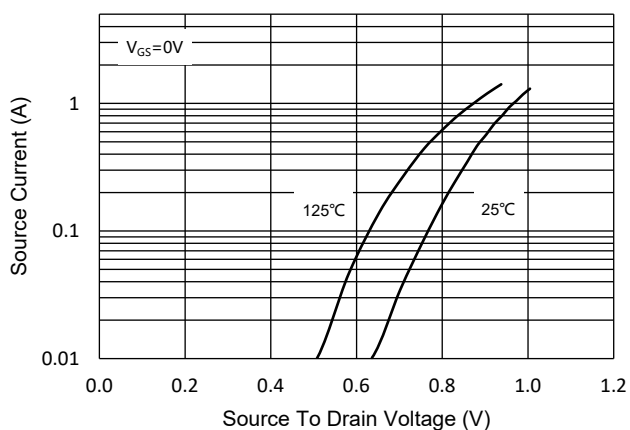
Fig.9 - I_S - V_{SD}
