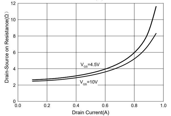
Fig. 4 - R_{DS(ON)} — I_D
