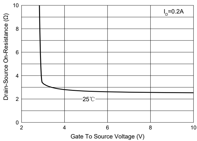
Fig. 3 - R_{DS(ON)} — V_{GS}
