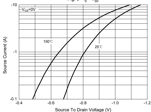
Fig. 9 - I_S - V_{SD}
