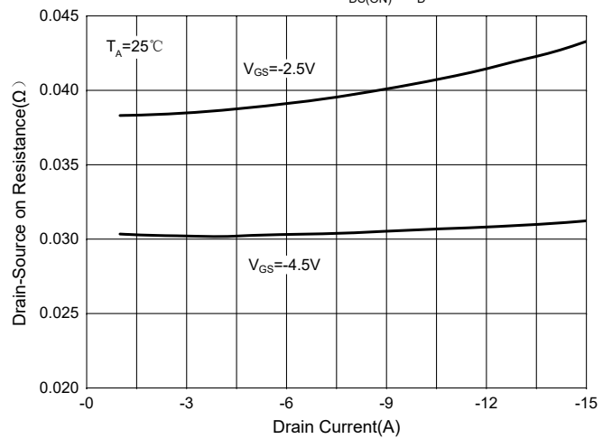
Fig. 4 - R_{DS(ON)} - I_D
